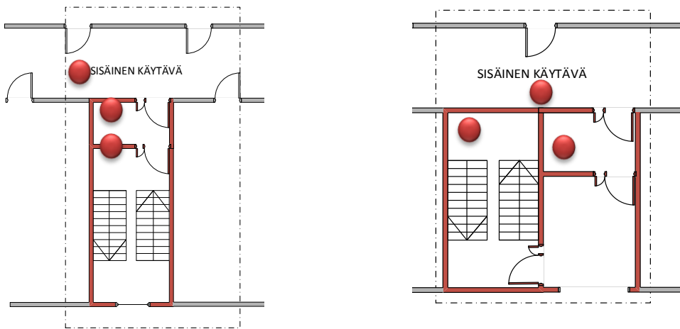
Kuva 66. Kuvassa vasemmalla on palolta suojattu uloskäytävä, oikealla on palolta ja savulta suojattu uloskäytävä (Kuikka). Punaiset pisteet kertovat missä nousujohdon ulosotto voi sijaita.
