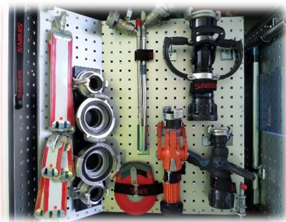
Kuva 11. Vasemmalla armatuuriikalustoa, oikealla vaahtokalustoa (Pelastusopisto).
