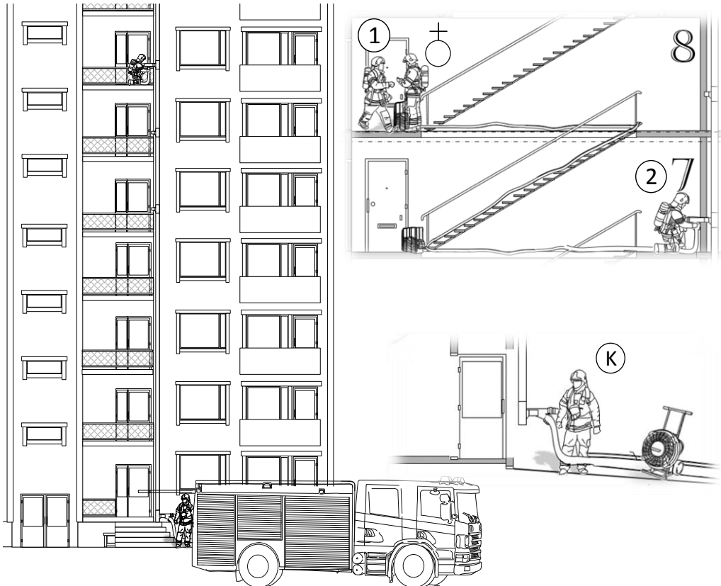
Kuva 33. Perusselvitys kerrokseen nousujohdolla. Nousujohdon sijainti ei ole rakennuksen ulkopuolella vaan sisällä. Tässä kuvassa se on piirretty ulkopuolelle havainnollistamaan selvitystä paremmin. (Kuikka.)
