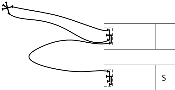
Kuva 42. Säiliöautoselvitys säiliösarjakytkennällä ilman vuoroliitintä (Kuikka).
